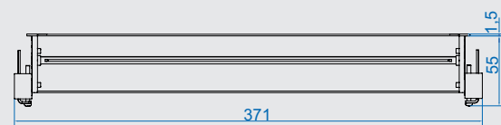
Rama montażowa VENID | Wymiary w mm
